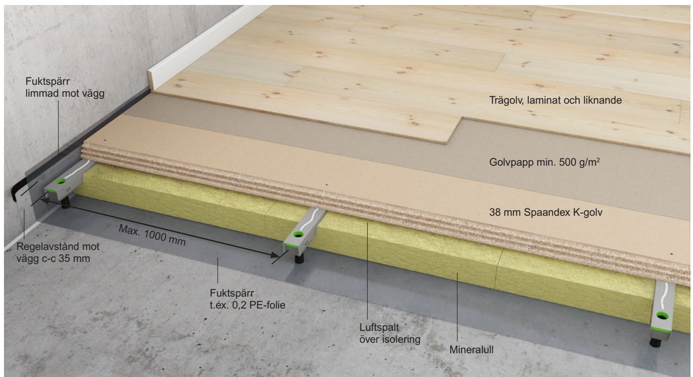
Figur 2 38 mm Spaandex K-golv på stålreglar. Regelavstånd max. 900 mm när skivorna stöds över regler. Regelavstånd max. 1000 mm när undergolvet är utfört utan understöd över skarvar (endast till allmänna bostäder med belastning max. 2 kN).
